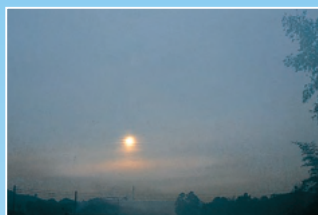
こうそううん 高層雲 (おぼろぐも)
