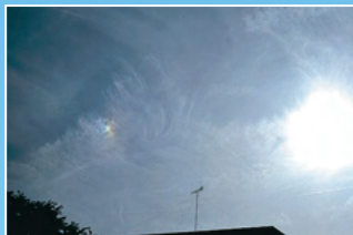
けんそううん 巻層雲 (うすぐも)
