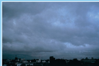
らんそううん 乱層雲 (あまぐも)
