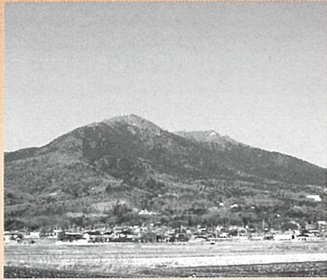
筑波山-7500万年前と6000万年前のマグマ-
