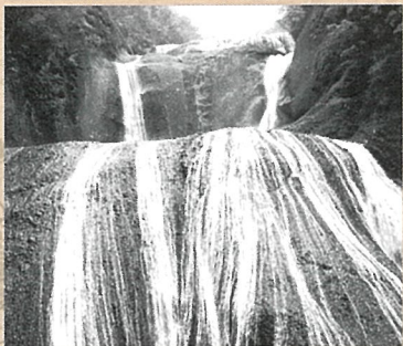
袋田の滝-1600万年前の海底火山-
